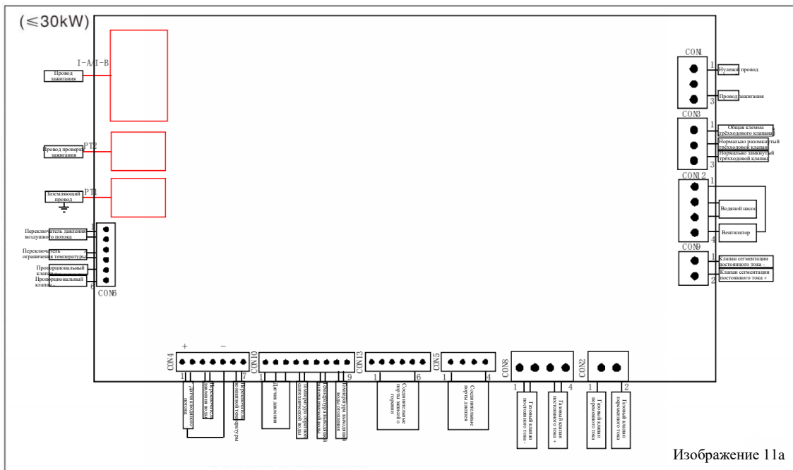
Схема с обозначениями проводов соединений системы газового настенного котла
